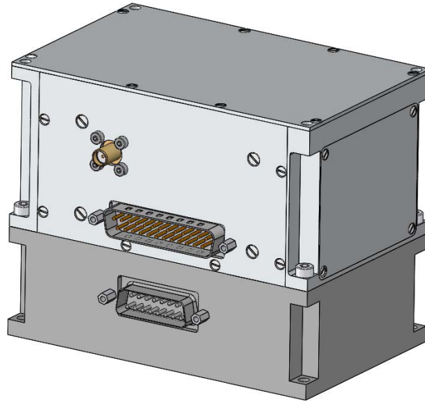
miniRAFS with OPTIONAL EPC module
